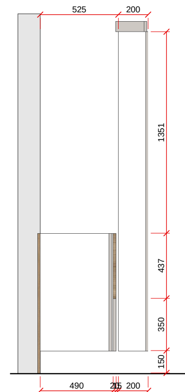
VISTA B - LATERAL - ESC. 1:25
