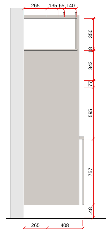
VISTA A - LATERAL - ESC. 1:25
