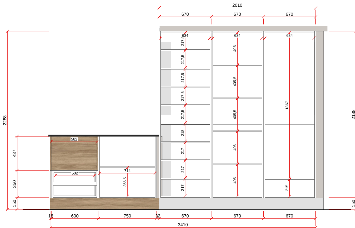
VISTA B - ESC. 1:25
